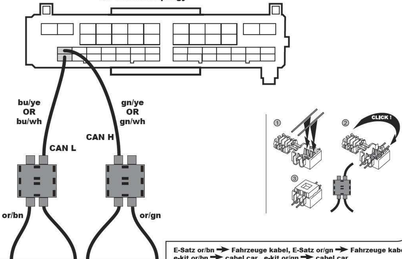
Fahrzeuge Stecker 50 pin gy car socket 50 pin gy
