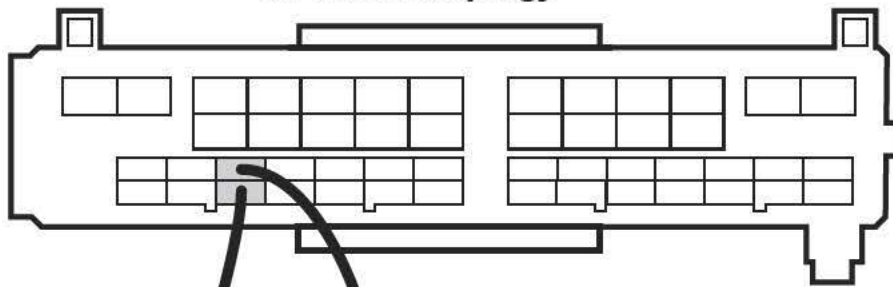
Fahrzeuge Stecker 50 pin gy car socket 50 pin gy
